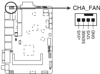
FAY-002 Fan connector
