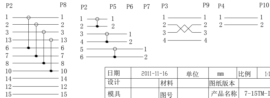
接线图
